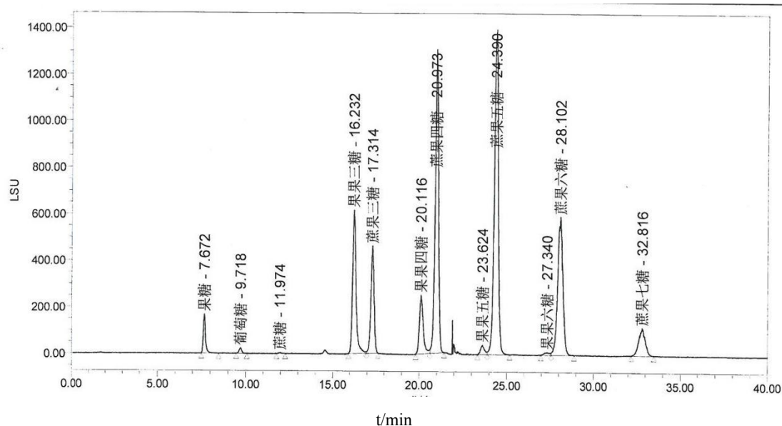
图 A. 2 氨基柱测定低聚果糖样品的谱图（高效液相色谱法参考条件 1）
