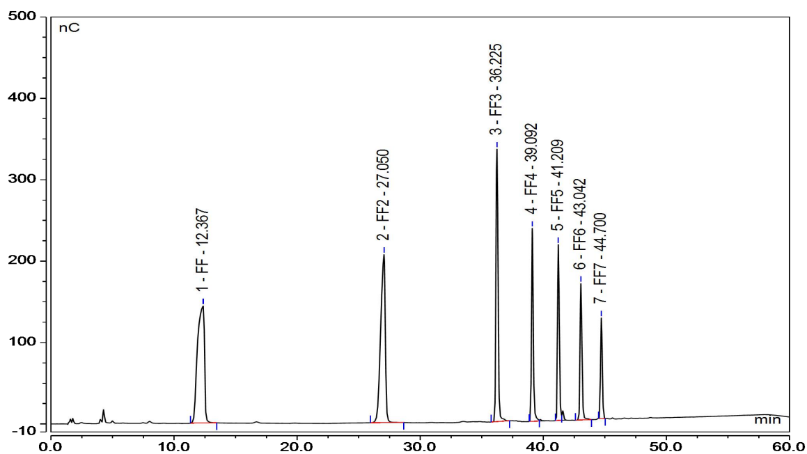
图 B. 3 6 个果-果型 (DP2-DP7) 糖组分的混合标样色谱图 (高效离子交换色谱法参考条件 1)
