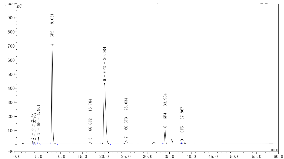
图 B. 4 测定蔗糖来源低聚果糖样品色谱图 (高效离子交换色谱法参考条件 1)
