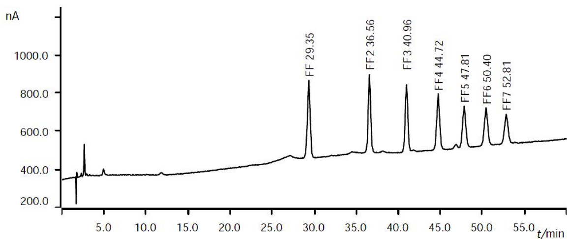
图 B.8 7 个果-果型 (DP2-DP7) 糖组分的混合标样色谱图 (高效离子交换色谱法参考条件 2)
