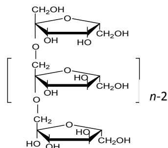
图 2 果-果型 ( F_n ) 低聚果糖分子结构示意图
