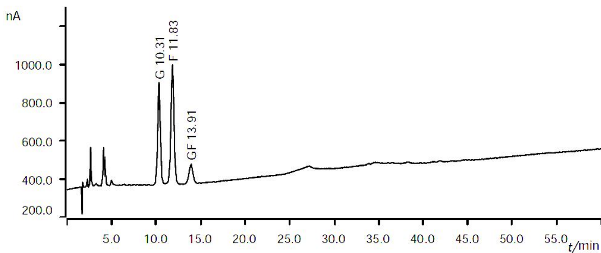
图 B.6 葡萄糖、果糖和蔗糖的混合标样色谱图（高效离子交换色谱法参考条件 2）
