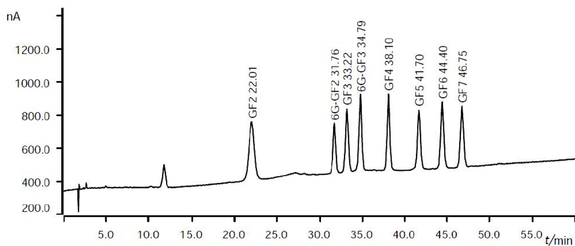
图 B.7 8 个蔗-果型 (DP3-DP7) 糖组分的混合标样色谱图（高效离子交换色谱法参考条件 2）
