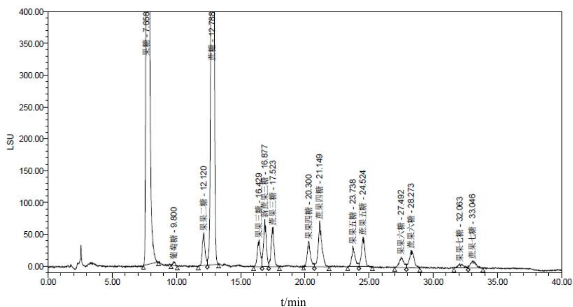
图 A. 1 氨基柱测定低聚果糖标准品的谱图（高效液相色谱法参考条件 1）
