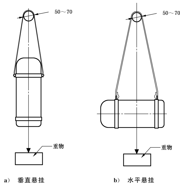
图 E.1 背带强度试验示意图
