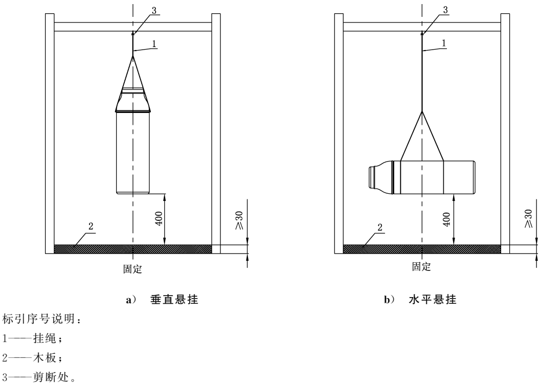
图 B.1 坠落冲击试验示意图
