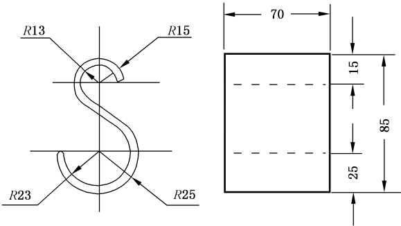
图 5 吊钩示意图
