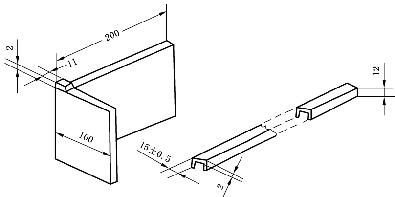
图 3 支架和搁条
